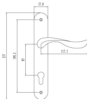
ALU.HANDLE REF.208W
