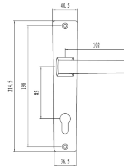
ALU.HANDLE REF.207B
